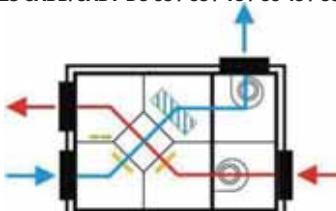
MODELES CADB/CADT-DC 05 / 08 / 18 / 30 / 45 / 56 GH DP
